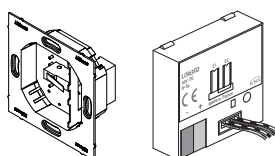
Li56302 : KNX Interface (2 buttons) Li56304 : KNX Interface (4 buttons)
